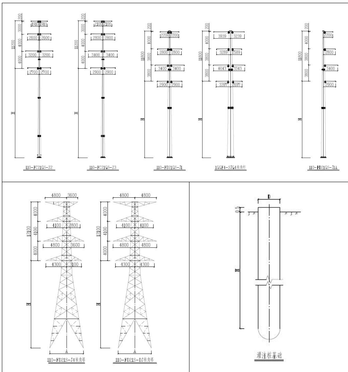
图 1.1-2 塔基型号及基础示意图
