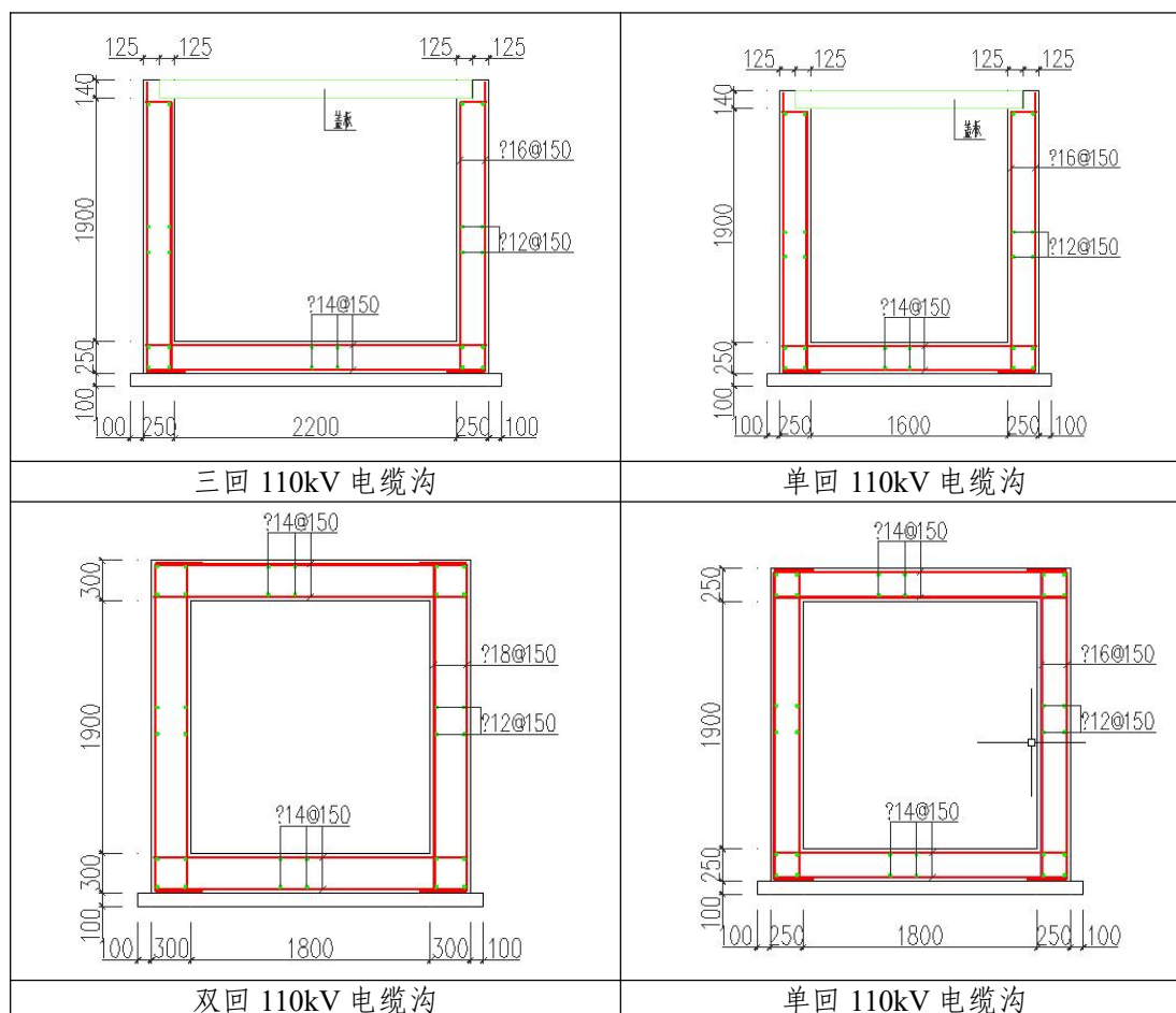
图 1.1-4 电缆沟断面图
