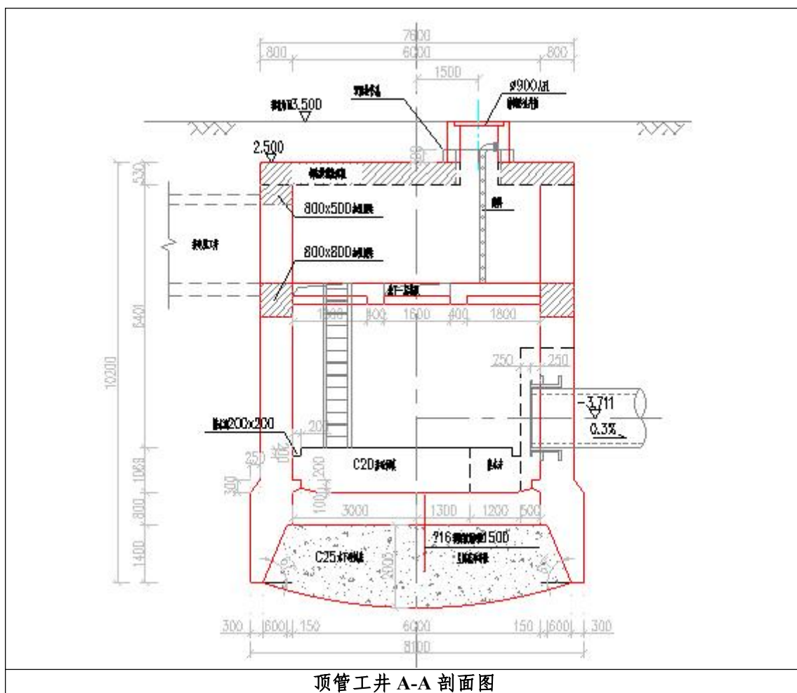
图 1.1-6 拉管和顶管平、剖面图
