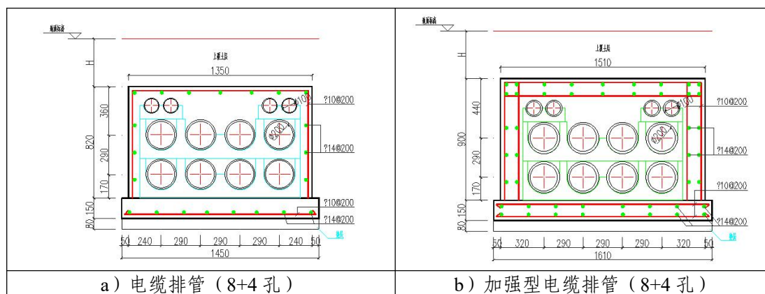
图 1.1-3 电缆排管断面图
