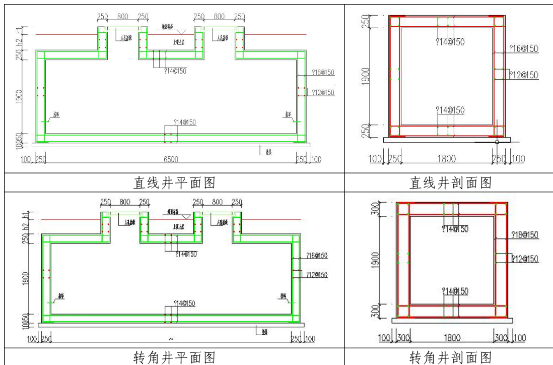
图 1.1-5 电缆井平、断面图
