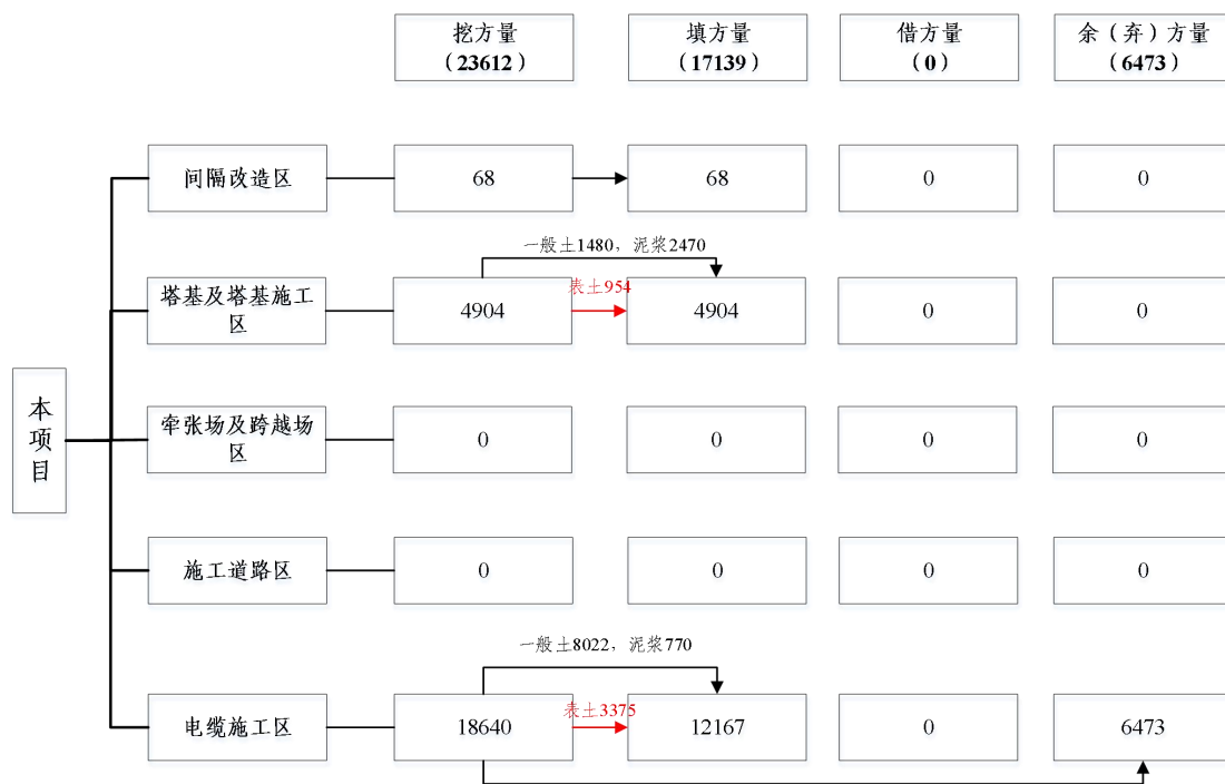
图 1.1-6 总土石方挖填平衡流向框图 (单位: m³)
